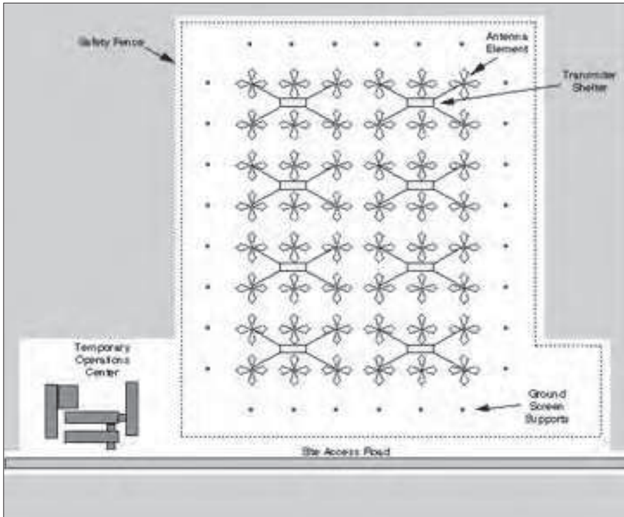
HAARP-Lageplan
